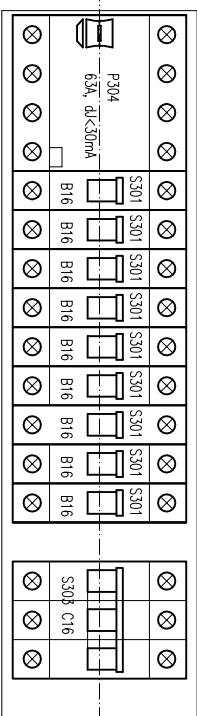
Tablica włączkowa typu Ekinox® TX 4 x 18 mod izolacyjnie, białe wymiary 760 x 425 x 133 mm wymiary wnętrza 710 x 410 x 100 mm
